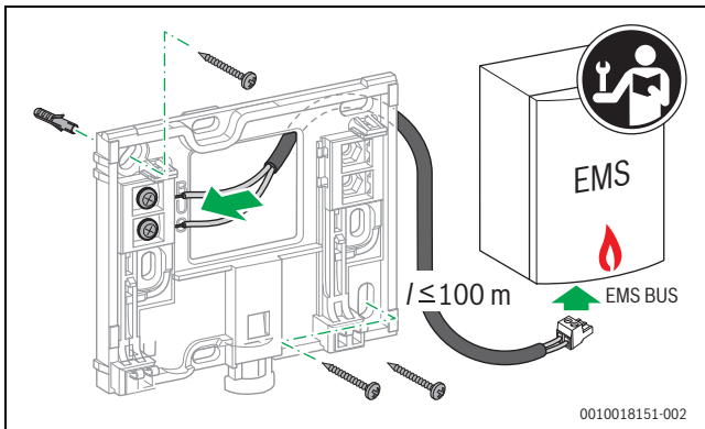
Afb. 5 Aansluiten sokkel
