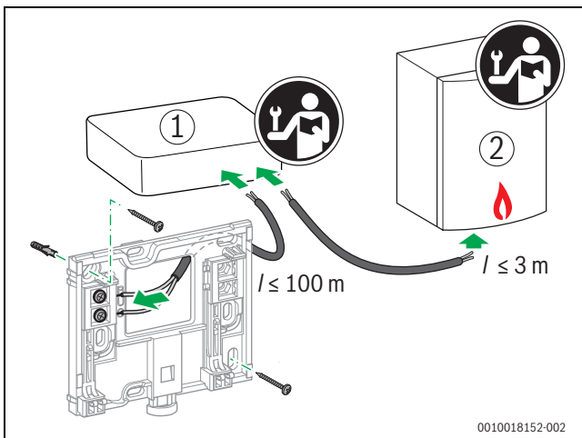
Afb. 6 Aansluiten van de EasyControl-adaptor
