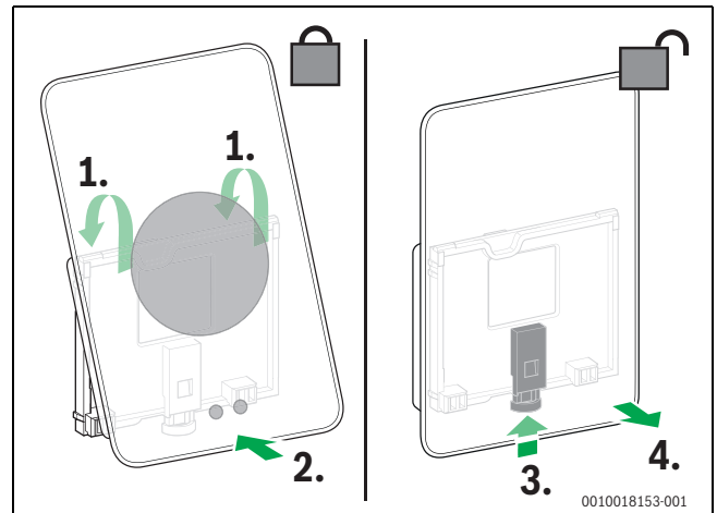
Afb. 7 (De)monteren regelaar
