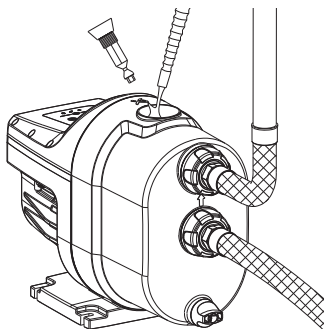
Amorçage du surpresseur
