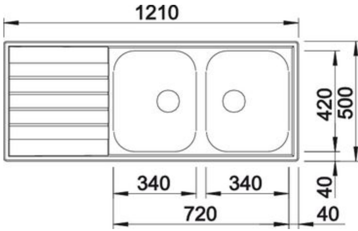
Bovenaanzicht
