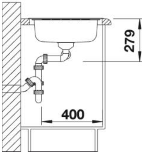
Zijaanzicht
